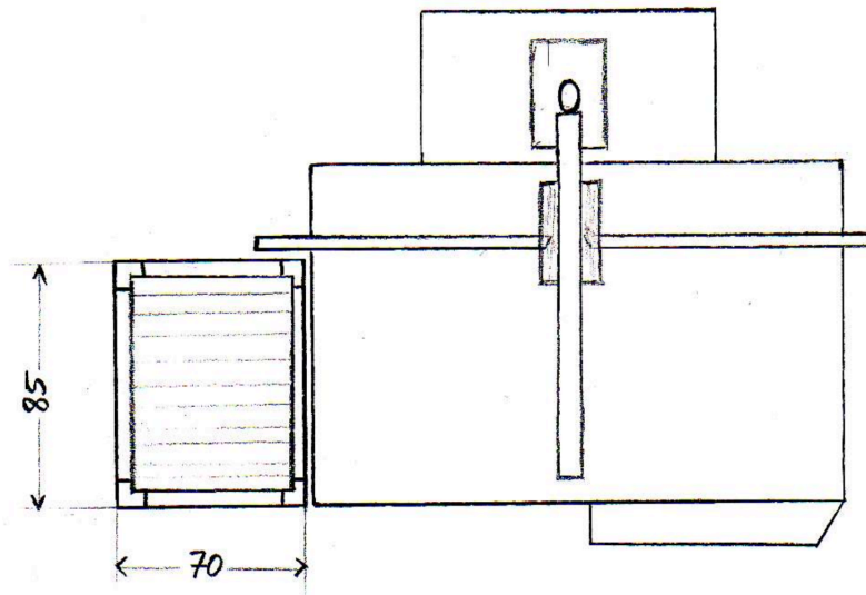
Croquis du bac à côté de la scie radiale (vue de dessus, échelle 1/20)
